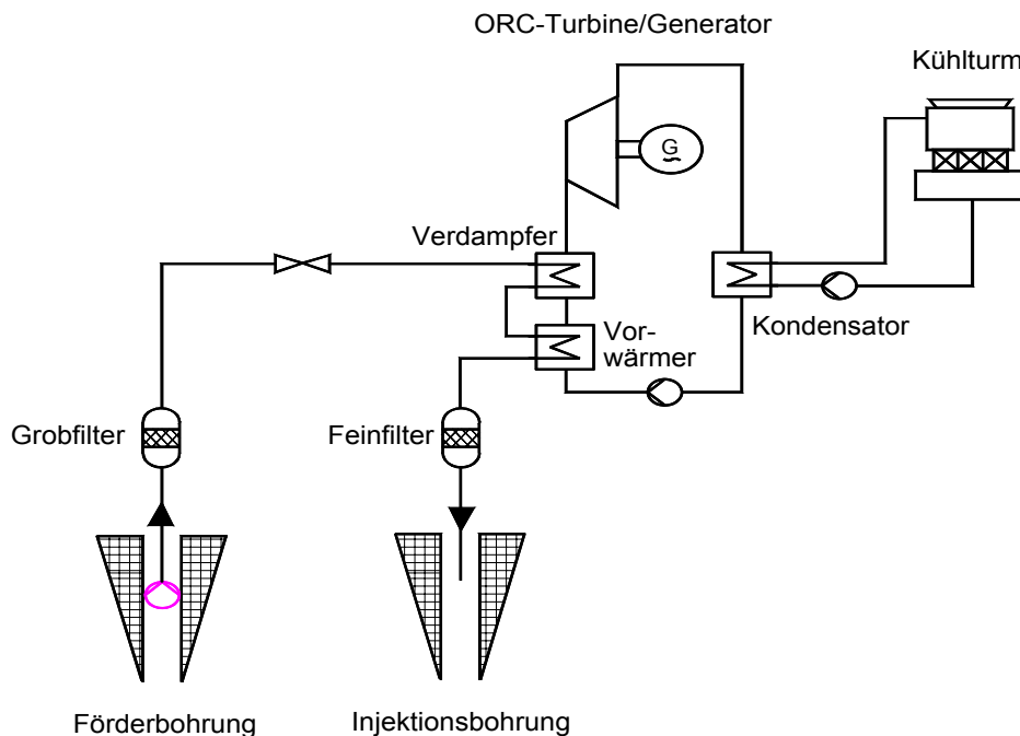
Abb. 21: Vereinfachtes Schema einer ORC-Anlage
