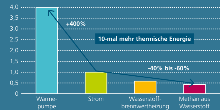
Abbildung 6: Nutzbare thermische Energie aus elektrischer Energie, Vergleich Erdwärmepumpe zu Wasserstoff aus Elektrolyse bzw. anschließender Methanisierung (Quelle: Eigene Darstellung, Annahmen Wirkungsgrade: Elektrolyse: 65%, Methanisierung: 80%, Kompression: 85%, Heizung: 90%). 7
