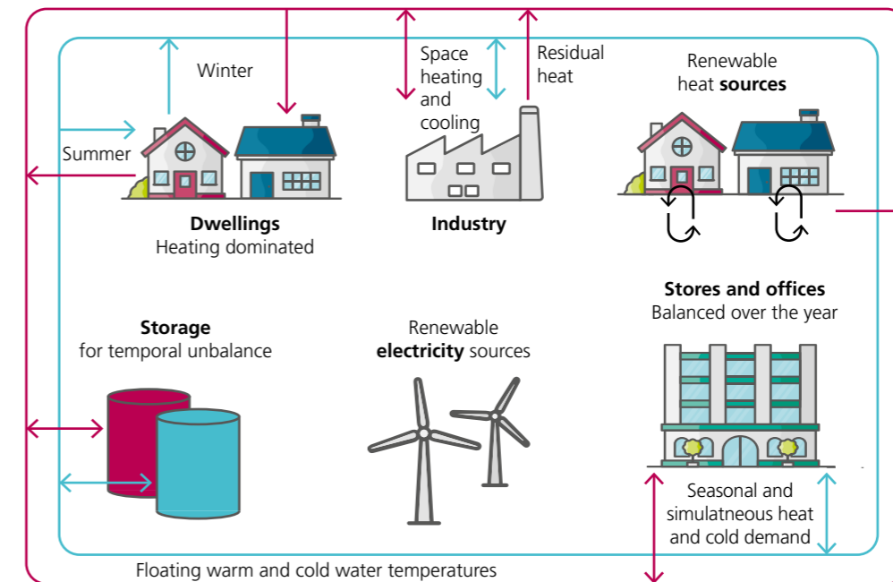
Abbildung 16 – Wärme- und Kältenetz der 5. Generation 24
