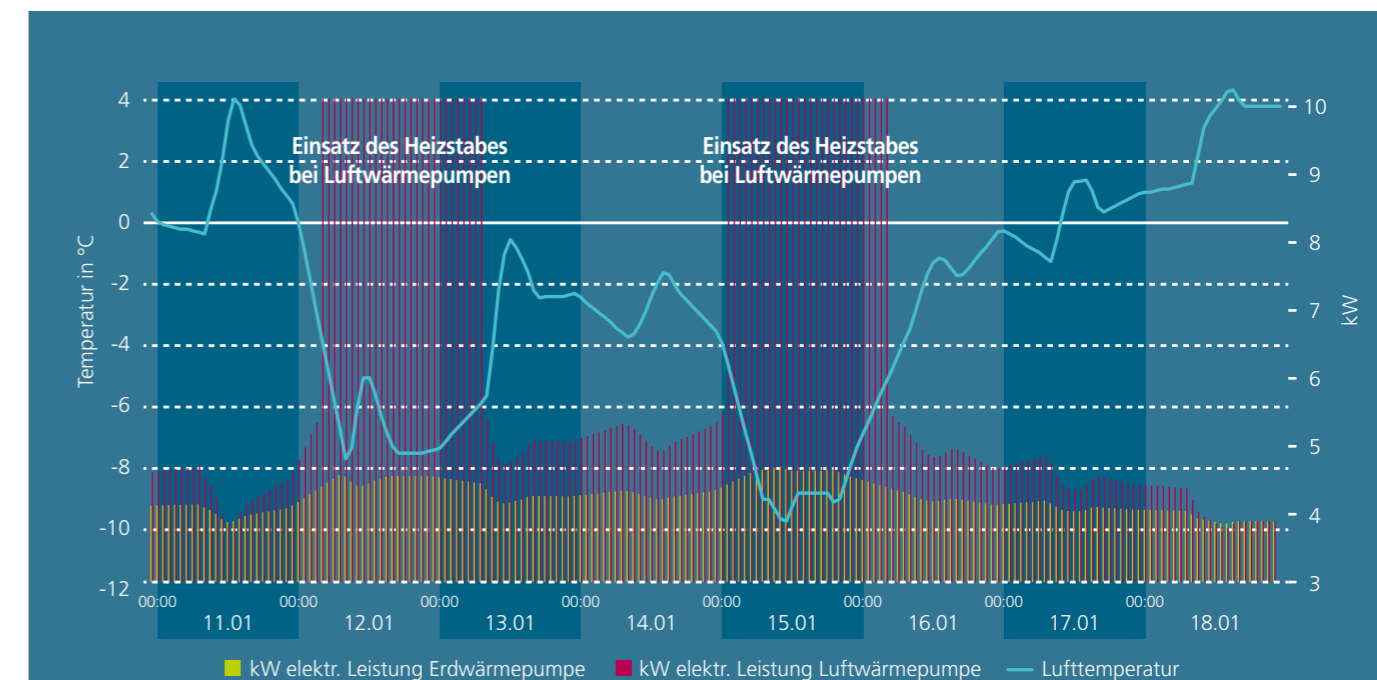
Abbildung 13 - Elektrische Lastspitzen bei Luftwärmepumpen durch den Einsatz des Heizstabes (Eigene Darstellung) 21
