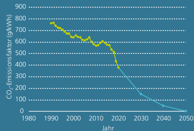
Abbildung 14 – CO 2 -Emissionen des deutschen Strommixes (Eigene Darstellung) 23
