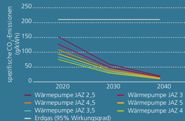
Abbildung 15 – CO 2 -Emissionen von Wärmepumpen in Abhängigkeit der JAZ (Eigene Darstellung)
