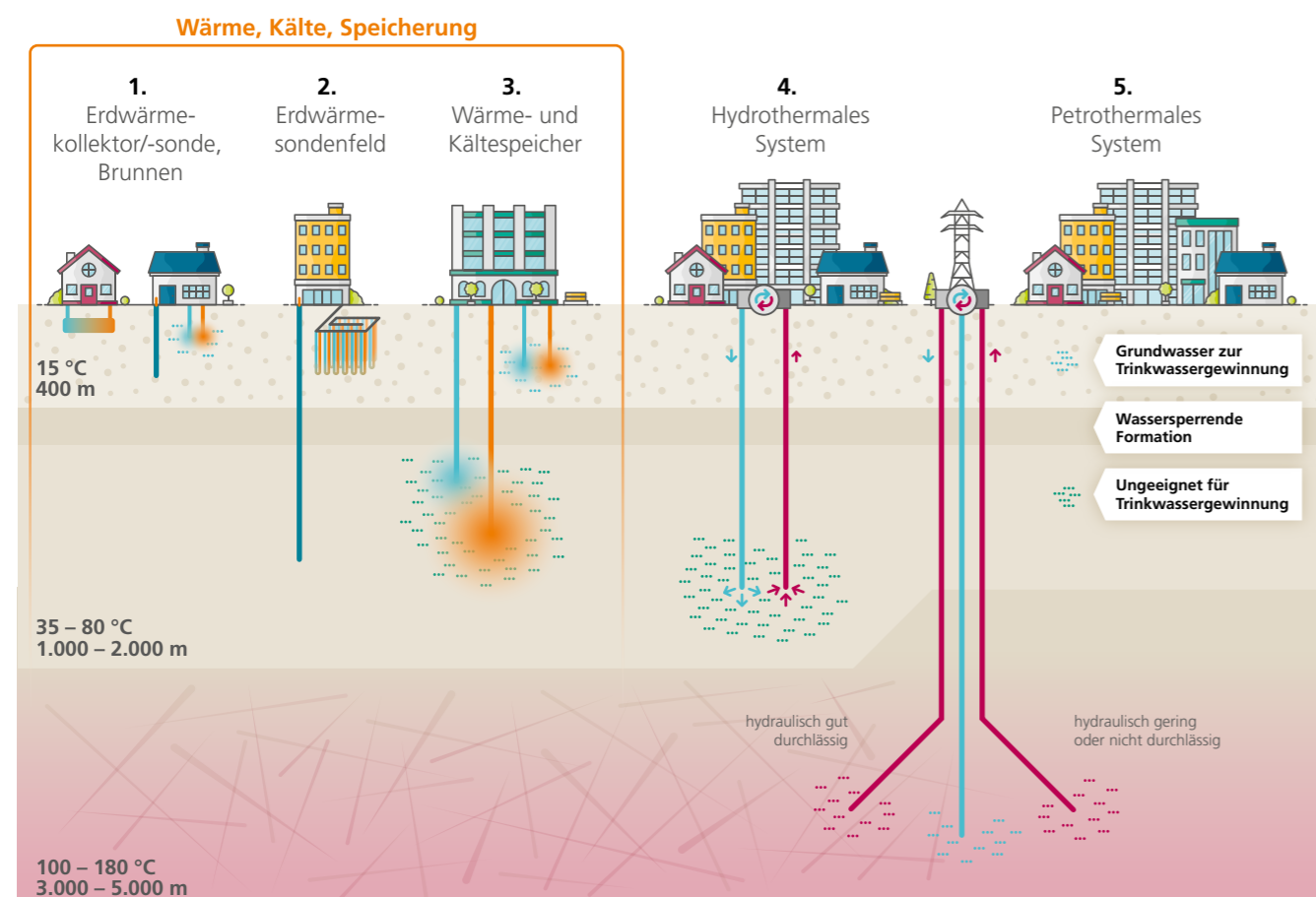
Abbildung 3: Erdwärmesysteme: Erdwärmesonden / Erdwärmekollektoren / Grundwasserbrunnen zur Gewinnung und Speicherung Wärme und Kälte aus oberflächennahen geologischen Formationen bis 400 m (Varianten 1 bis 3) für Einzelobjekte und die Quartiersversorgung (Gegenstand dieses Papiers). Tiefengeothermische hydrothermale und petrothermale Systeme (Varianten 4 und 5) reichen bis in 5.000 m Tiefe und werden für großtechnische Anwendungen genutzt.
