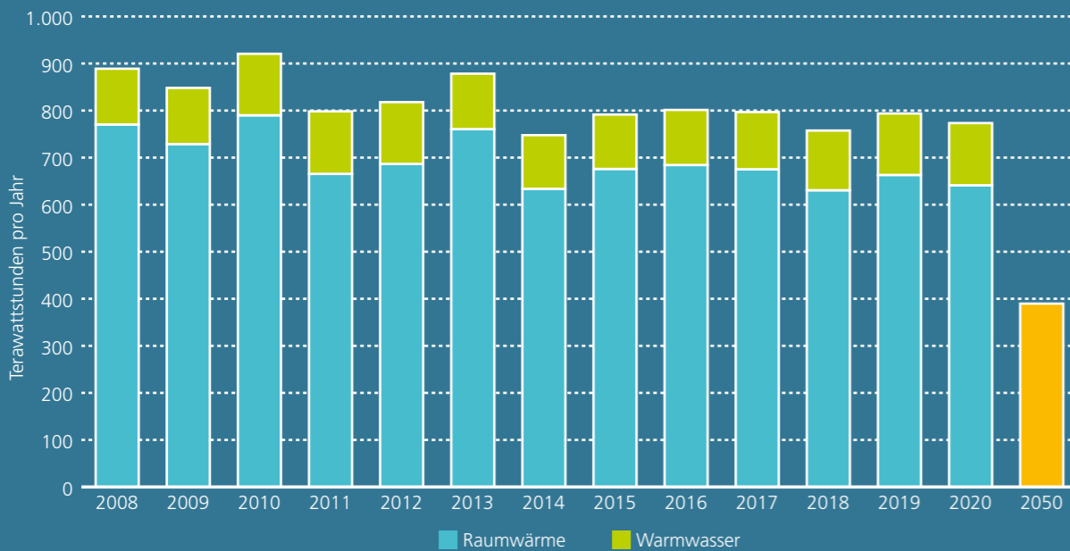
Abbildung 1: Nutzwärmebedarf (Raumwärme und Warmwasser) in Deutschland. Absoluter langjähriger Bedarf in TWh/a, Prognose 2050 (Eigene Darstellung). 1
